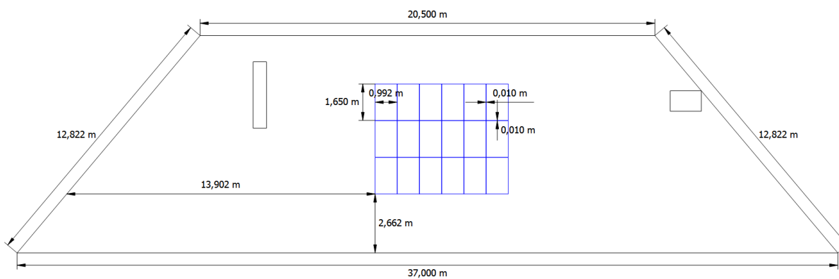
Rys. 6. Obszar posadowienia instalacji na zachodniej połaci dachu
