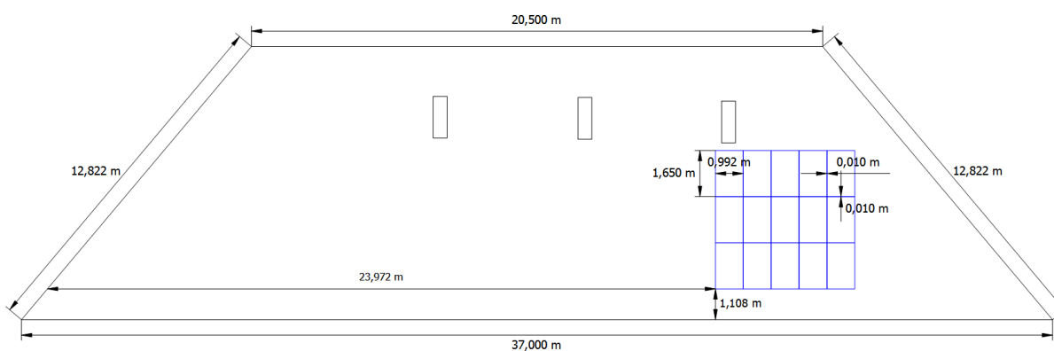
Rys. 4. Obszar posadowienia instalacji na południowej połaci dachu
