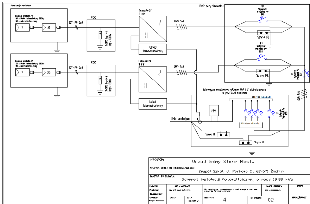
Rys. 3. Schemat jednokreskowy instalacji
