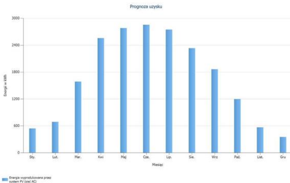
Rys. 10. Uzyski energii z instalacji fotowoltaicznej
