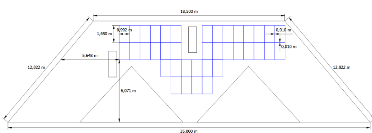
Rys. 4. Obszar posadowienia instalacji na południowej połaci dachu
