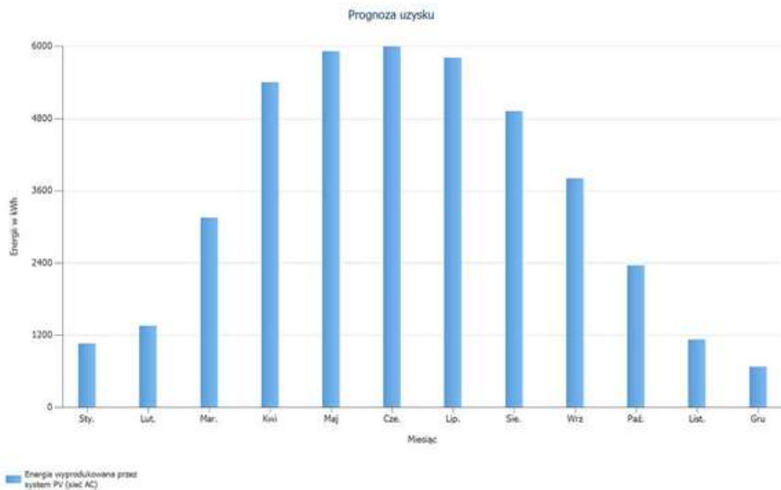
Rys. 7. Uzyski energii z instalacji fotowoltaicznej
